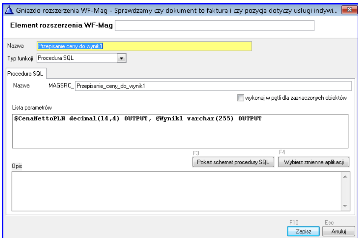
Rys. 43 Procedura przepisania ceny do zmiennej @Wynik1 (Przykład 4)
