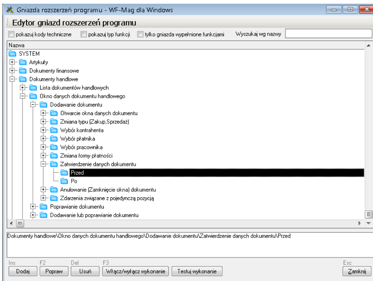
Rys. 3 Edytor gniazd rozszerzeń – w części dolnej widać adres gniazda
