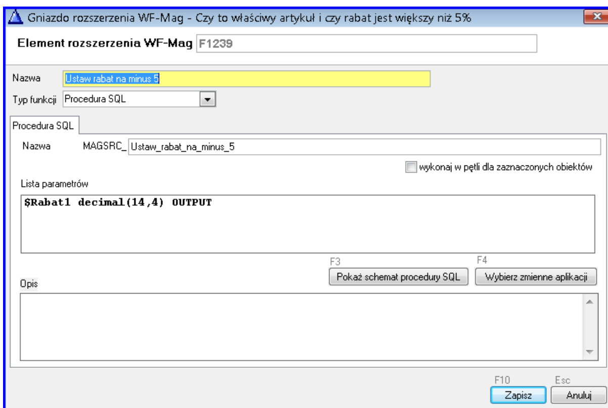
Rys. 28 Definicja wywołania procedury SQL ustawiającej rabat na -5 (Przykład 3)
