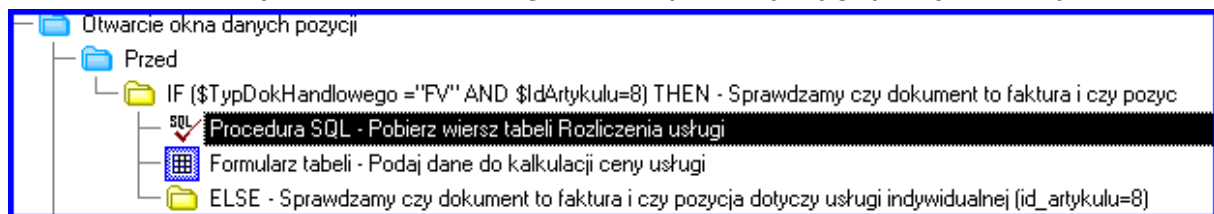
Rys. 38 Poprawna definicja wywołania formularza tabeli „Rozliczenie usługi” (Przykład 4)
