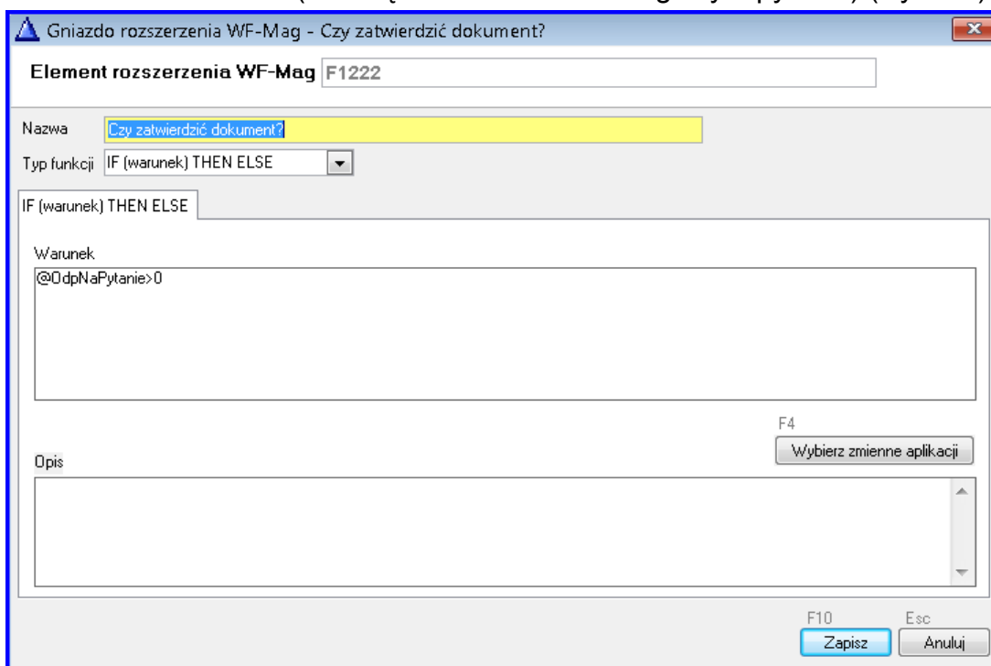
Rys. 22 Dodawanie funkcji IF (warunek) THEN ELSE (Przykład 2)
