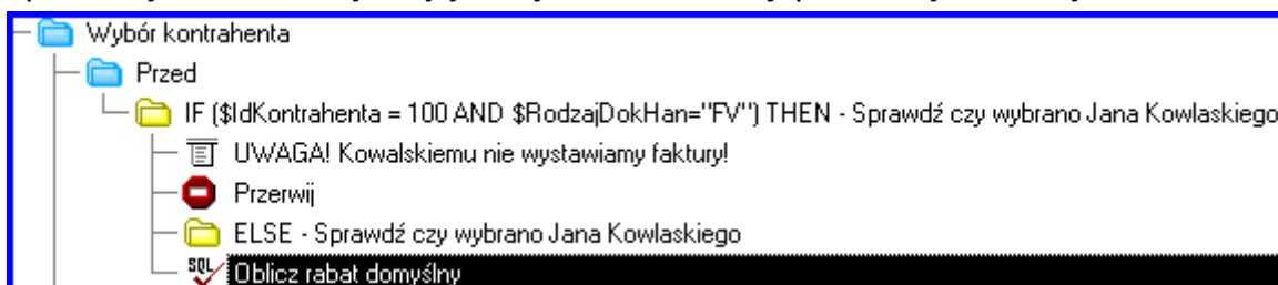
Rys. 10 Instrukcja warunkowego wykonania – funkcja na tym samym poziomie co ELSE
