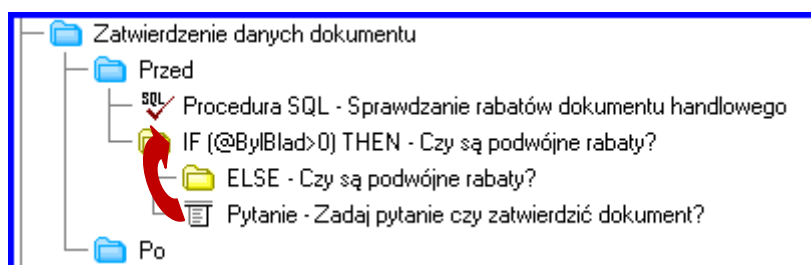
Rys. 20 Przeniesienie Pytania przed ELSE (Przykład 2)
