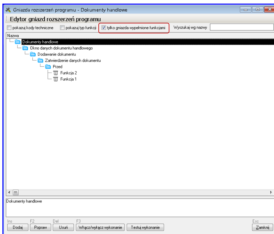
Rys. 13 Włączony filtr „tylko gniazda wypełnione funkcjami”
