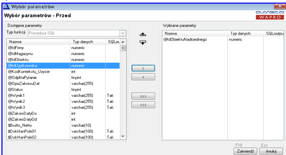
Rys. 5 Wybór parametrów dla procedury SQL
