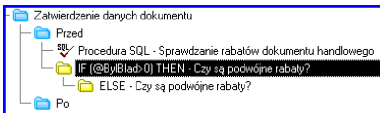
Rys. 18 Stan gniazda po dodaniu instrukcji IF (warunek) THEN ELSE (Przykład 2)
