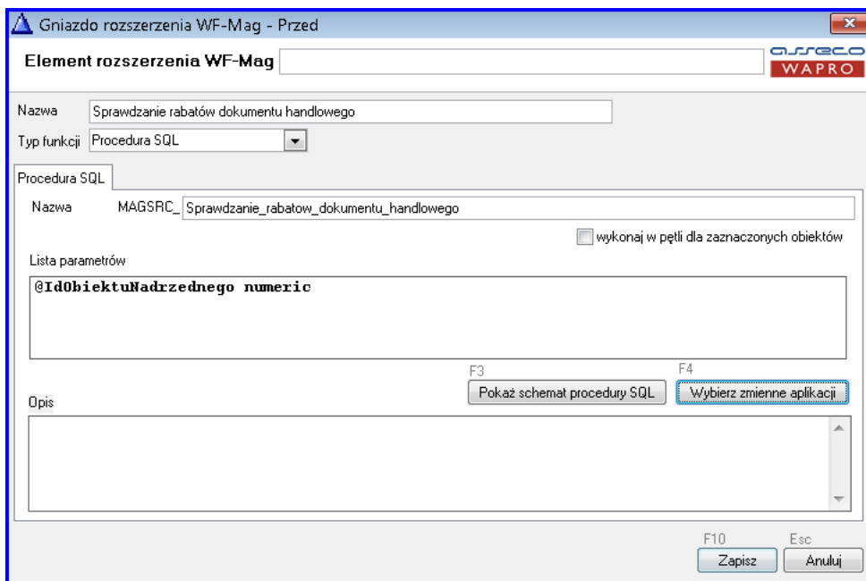
Rys. 14 Dodawanie funkcji typu Procedura SQL w gnieździe
