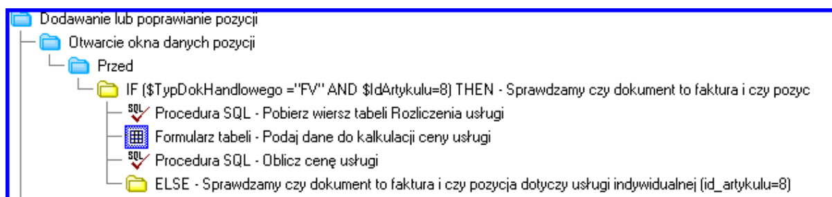
Rys. 40 Pobranie danych do kalkulacji ceny i jej obliczenie (Przykład 4)
