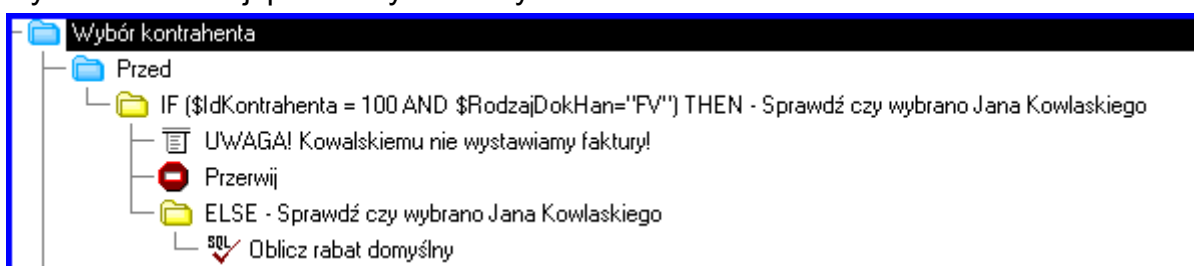
Rys. 9 Instrukcja warunkowego wykonania – funkcja podpięta do ELSE
