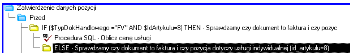
Rys. 42 Przy zatwierdzaniu danych pozycji trzeba sprawdzić cenę (Przykład 4)
