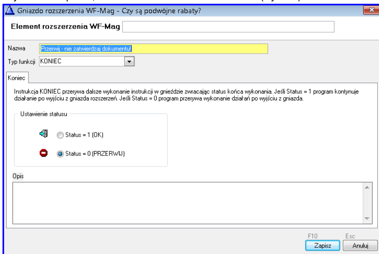
Rys. 24 Definiowanie funkcji Koniec z opcją Przerwij (Przykład 2)
