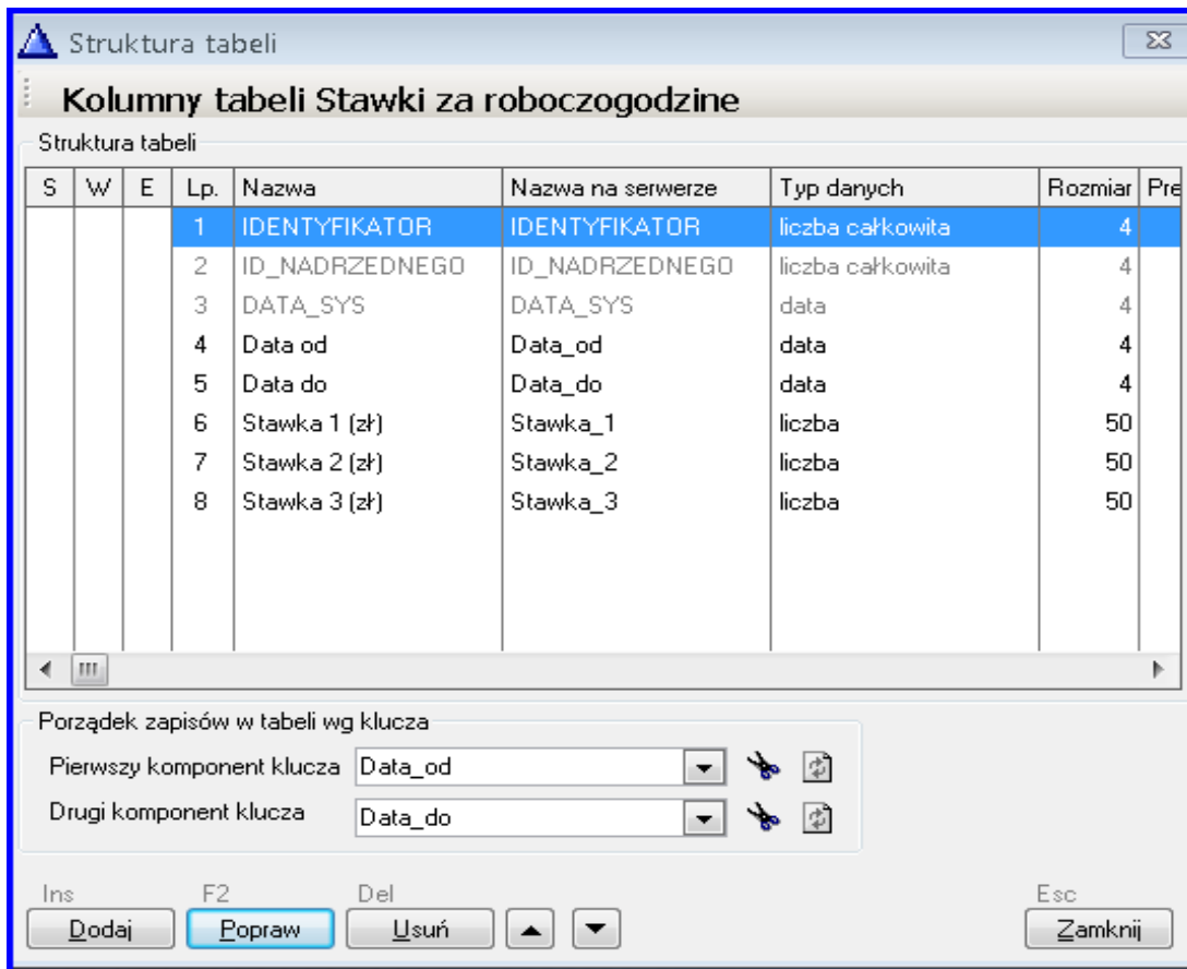
Rys. 32 Struktura tabeli „Stawki za roboczogodzinę” (Przykład 4)
