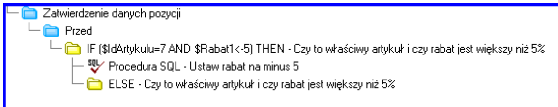
Rys. 29 Zawartość gniazda po dodaniu procedury SQL (Przykład 3)
