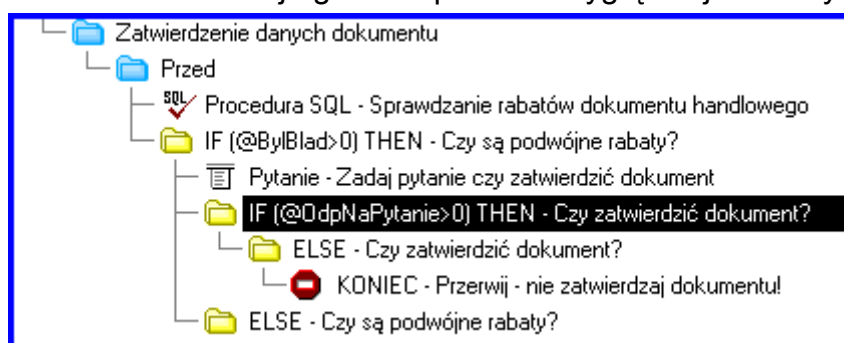
Rys. 25 Ostateczna postać definicji (Przykład 2)
