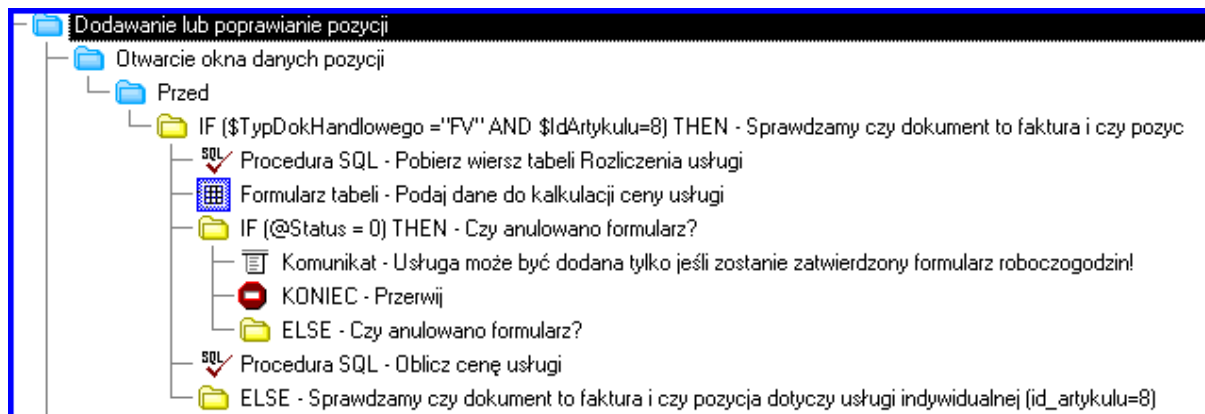
Rys. 41 Zawartość gniazda po dodaniu obsługi anulowania formularza (Przykład 4)
