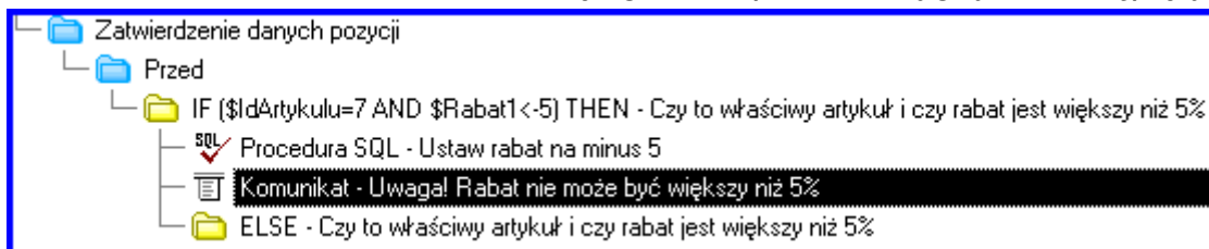
Rys. 31 Ostateczna postać definicji gniazda (Przykład 3)
