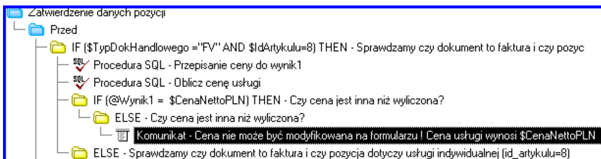
Rys. 44 Obsługa zatwierdzania pozycji (Przykład 4)
