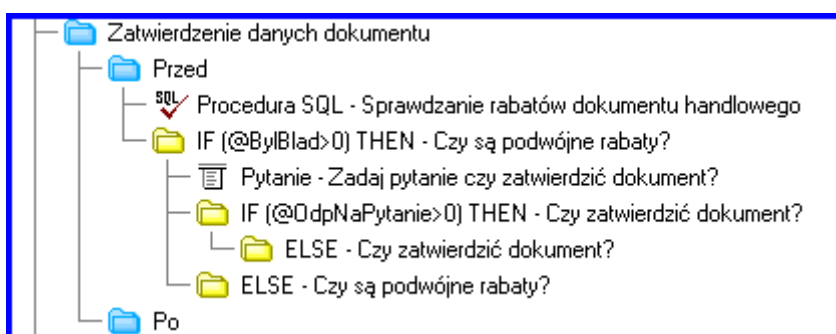
Rys. 23 Obsługa odpowiedzi na pytanie (Przykład 2)
